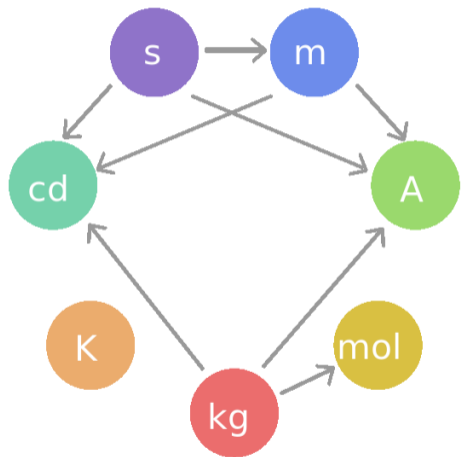
Abb. 1: SI Basiseinheiten [1]
