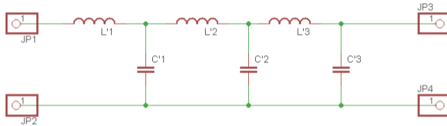
Abb. 2: Ersatzschaltbild
